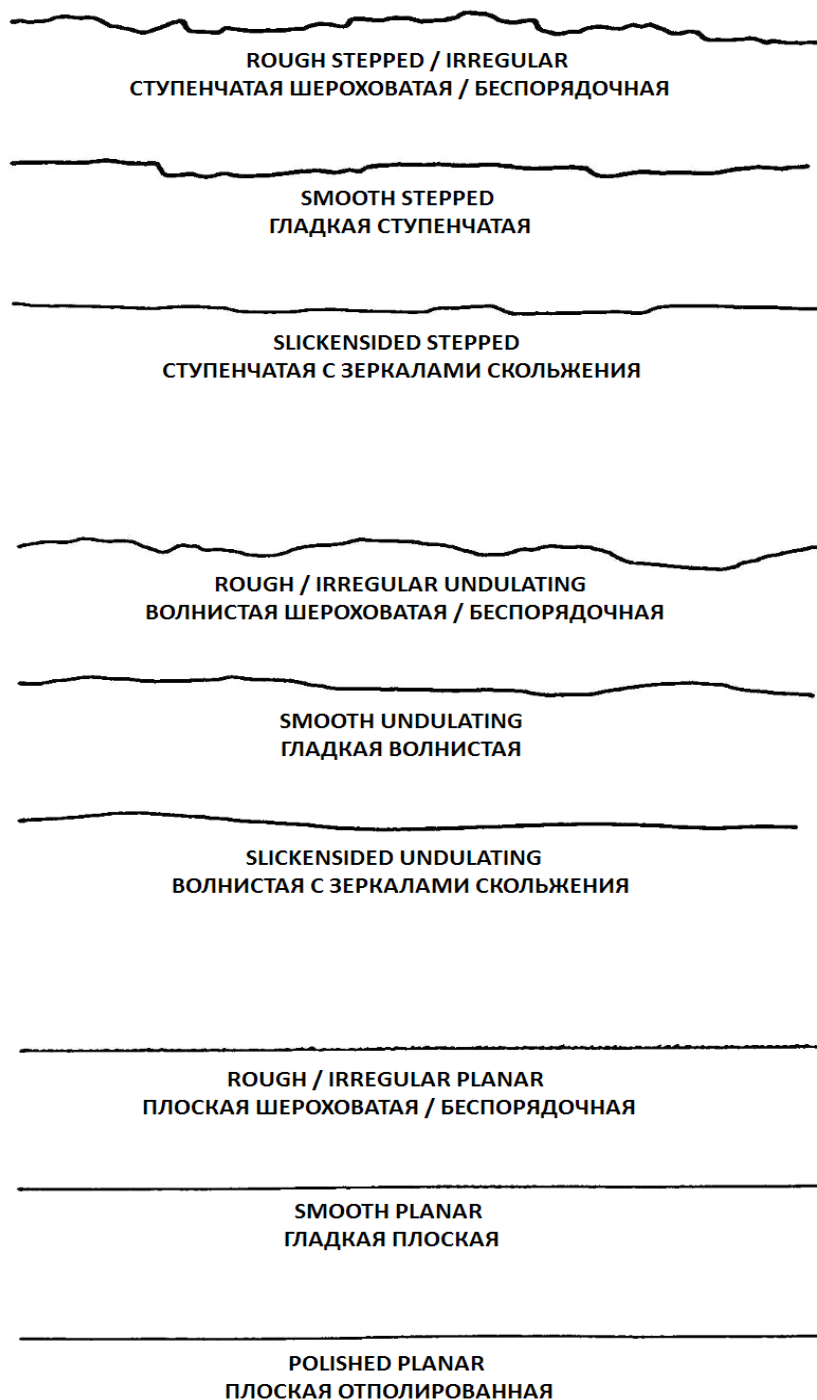
Рис. 15. Шаблон определения микрошероховатости.
