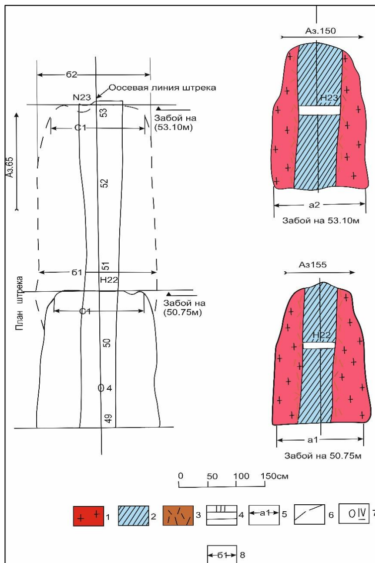
6-rasm. Zaboylar chizmalarini gorizonttal rejalar bilan bog‘lash misolidagi tasvir.
