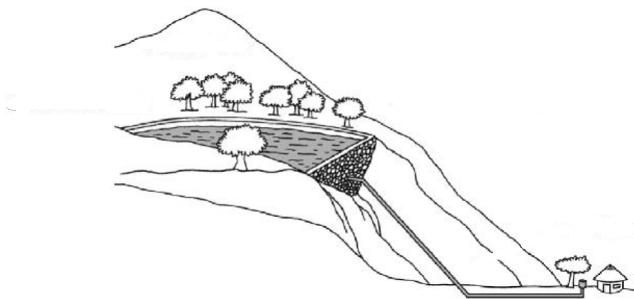
5-расм. Тошли тўғонлар
