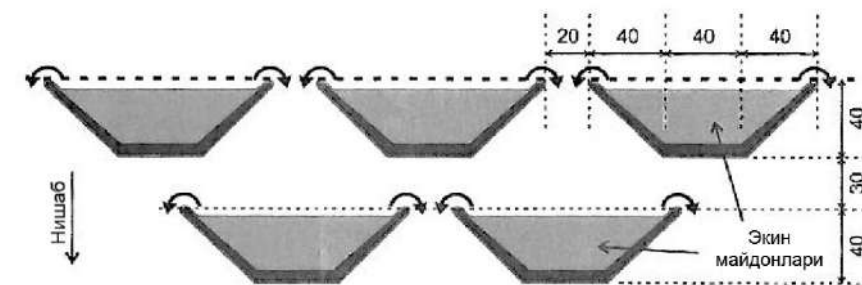
6-расм. Трапеция шаклидаги тўғонлар
