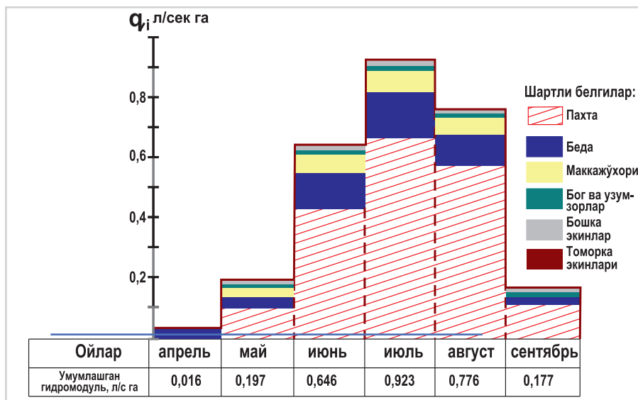
20-расм. Майдонда етиштириладиган экин турлари асосида умумлаштирилган гидромулдуль графиги
