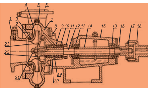
7-расм. Консолли турдаги марказдан қочма насоснинг тузилиши:
