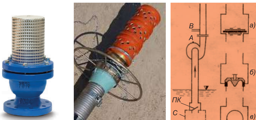
13-расм. Насосга сув тўлдириш учун қўлланиладиган қопқоқ:
