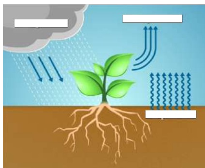
2-расм. Эвапотранспирация
