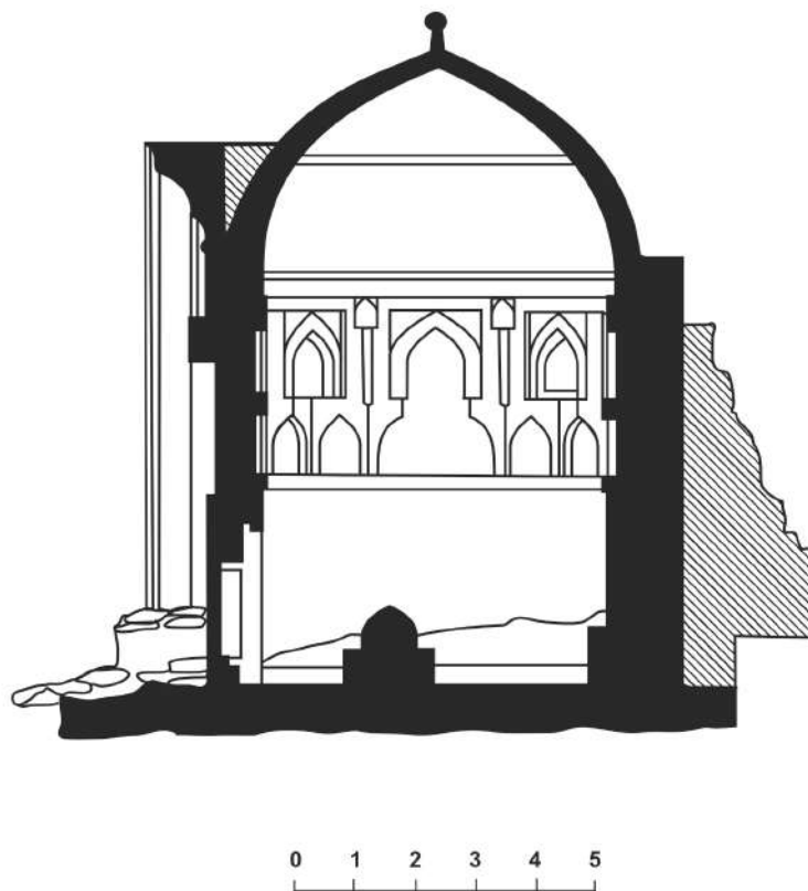
3-rasm. Maqbara qirgimi.
