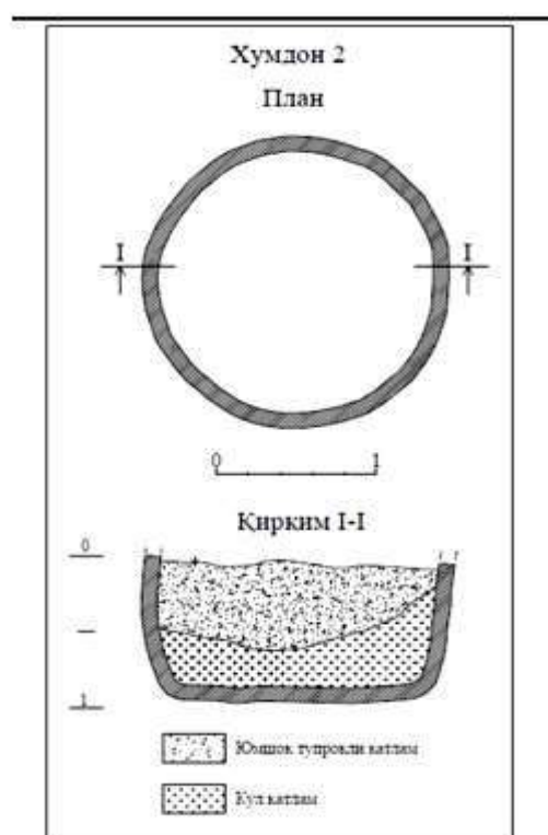
6-rasm. Changalli: Xumdon 2 ning umumiy ko‘rinishi, chizmasi va kesmasi.
