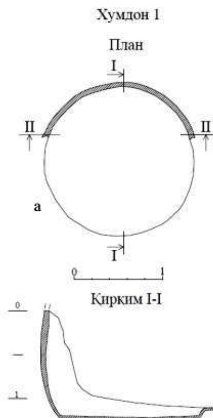
5-rasm. Changalli: Xumdon 1 ning umumiy ko‘rinishi, chizmasi va kesmasi.
