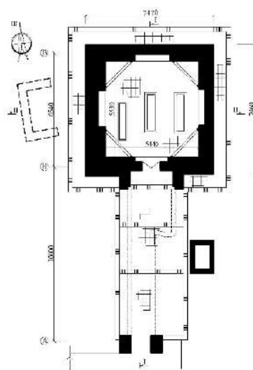
4-rasm. Ostona bobo maqbarasining rejasi. 1989-yil ta‘mirlash loyihasi materiallaridan
