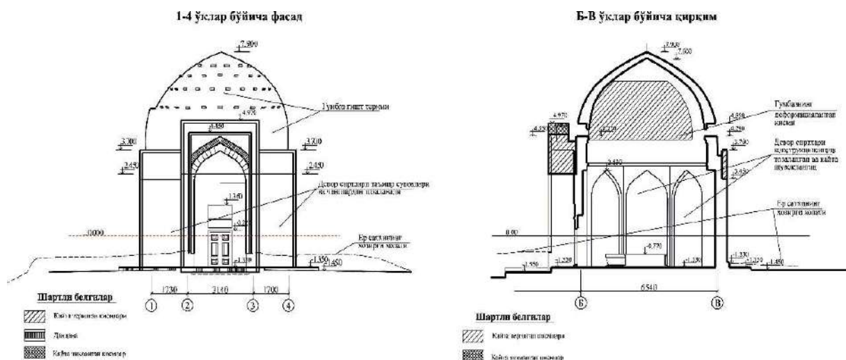
2-rasm. Ostonabobo maqbarasining janubiy, shimoliy tarzlari va qirqimi. 1989-yil ta'mirlash loyihasi materiallaridan.
