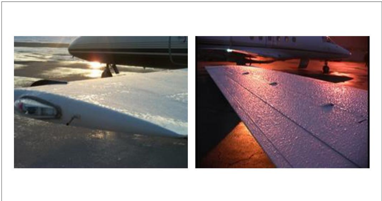
Рис. II-1-1. Примеры обледенения поверхностей самолета
