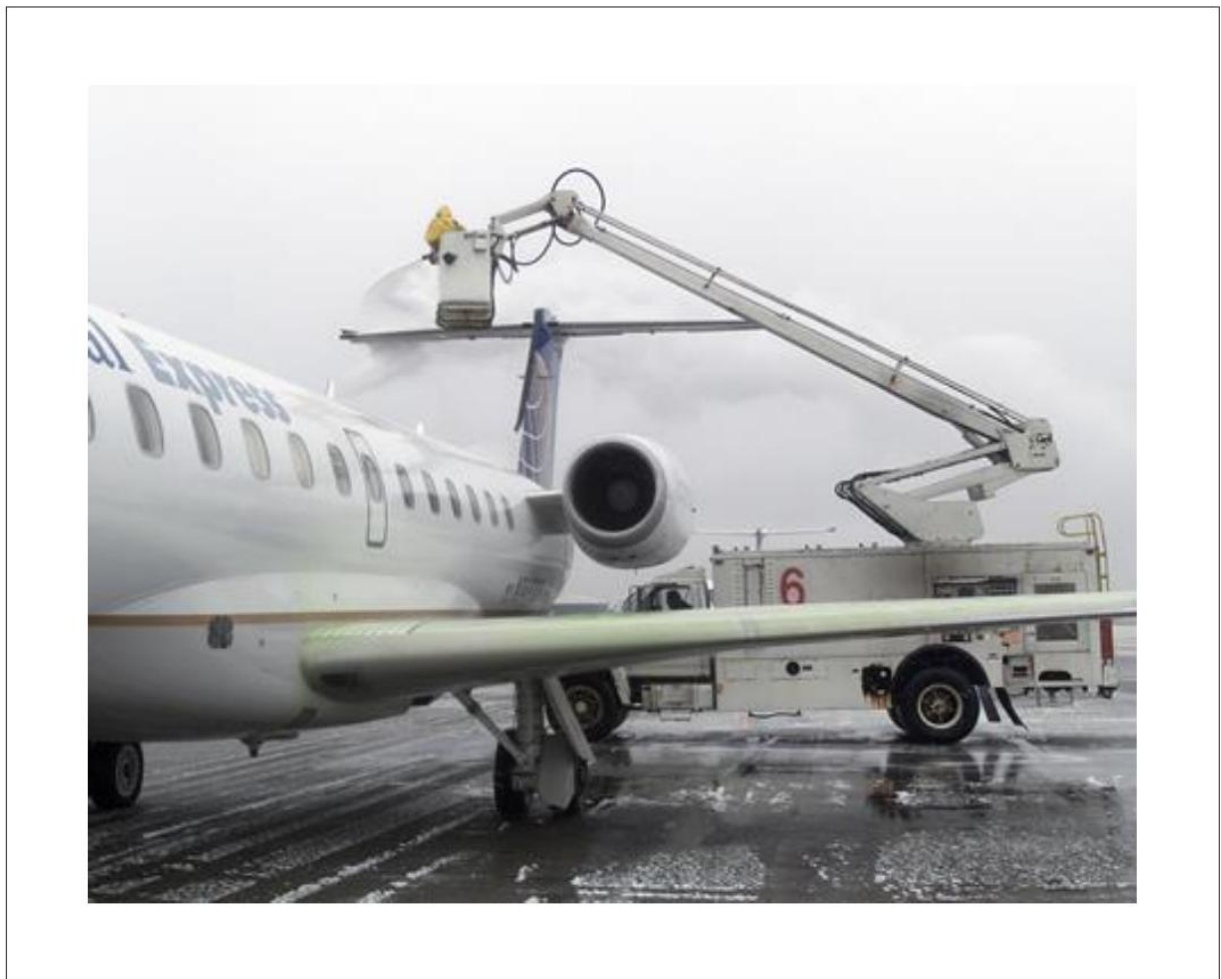
Рис. III-10-1. Типичное наземное противообледенительное оборудование
