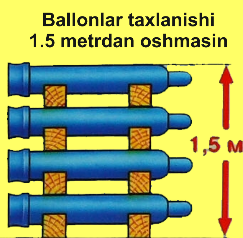
Ballonlar jo'mraklari bir tomonga qaratilgan bo'lishi shart
